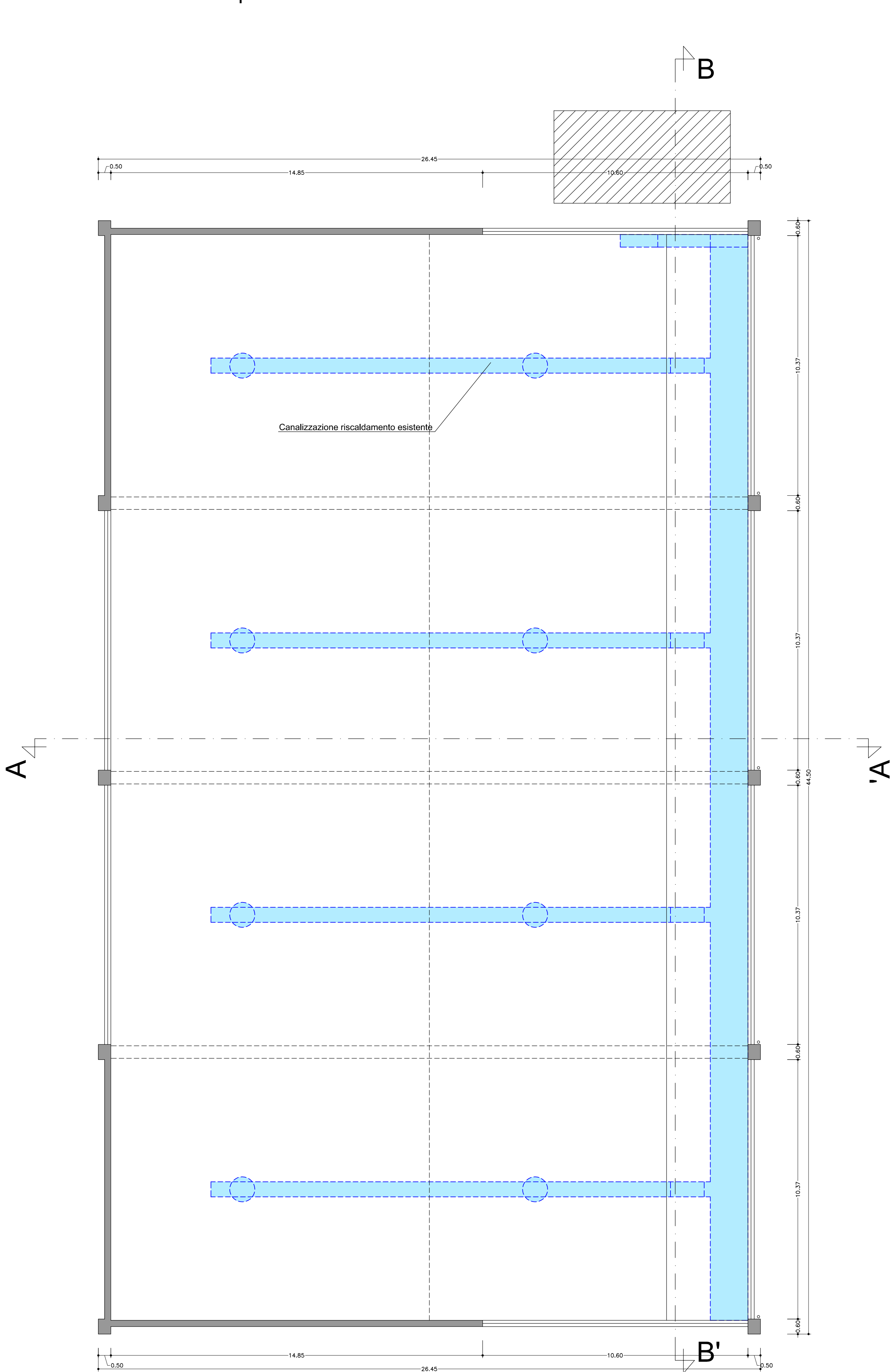
PIANTA - Livello finestratura palestra -
