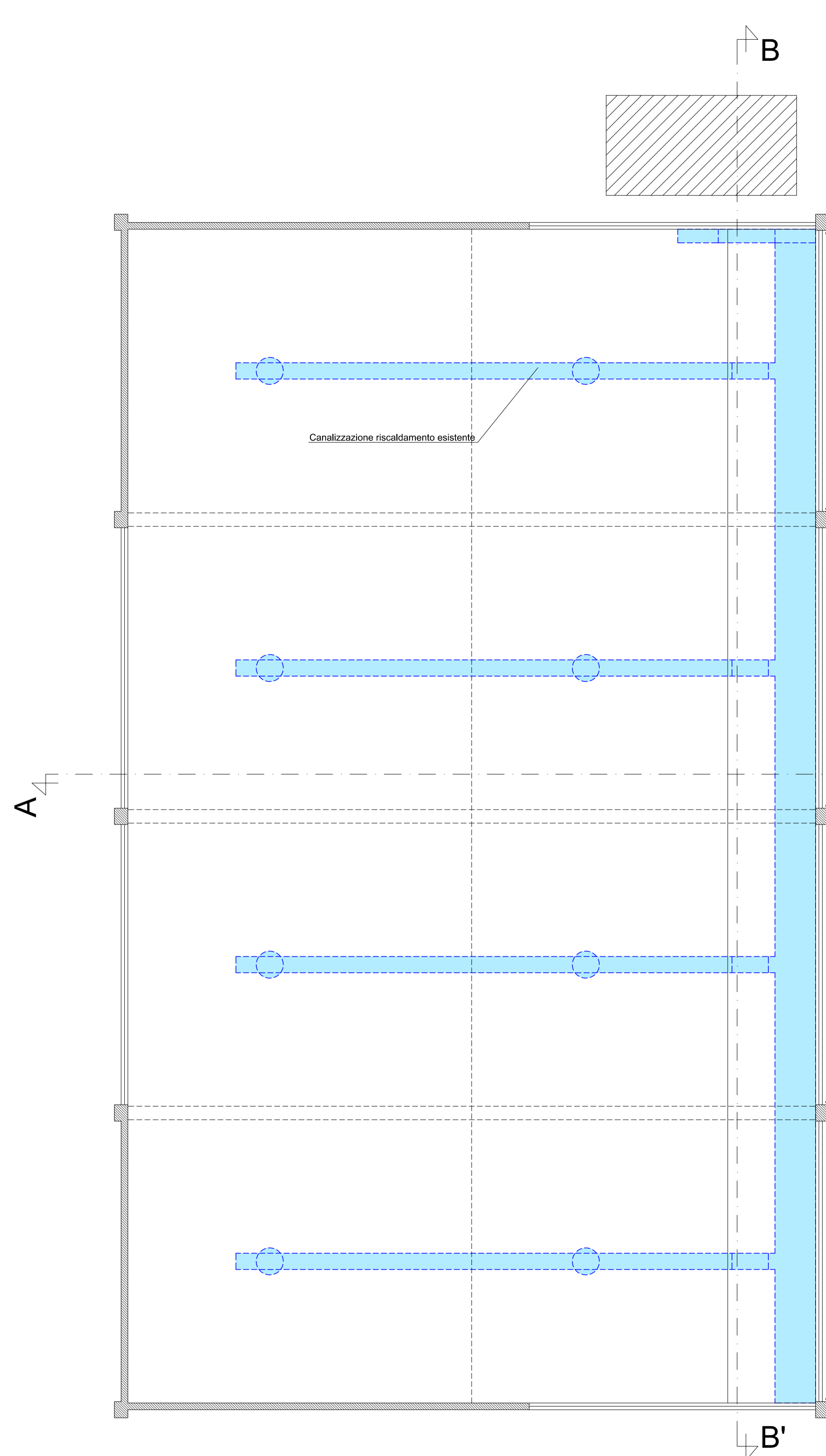
PIANTA - Livello finestrata palestra -
